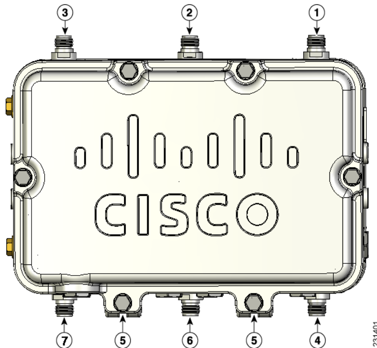
Figure 2 Emplacement des ports d'antenne
