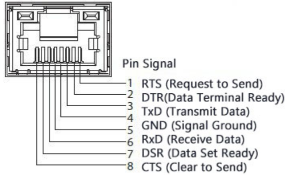
그림 20: 80-Series 및 90-Series 하드웨어에서 시리얼 포트에 대한 핀아웃 세부사항
