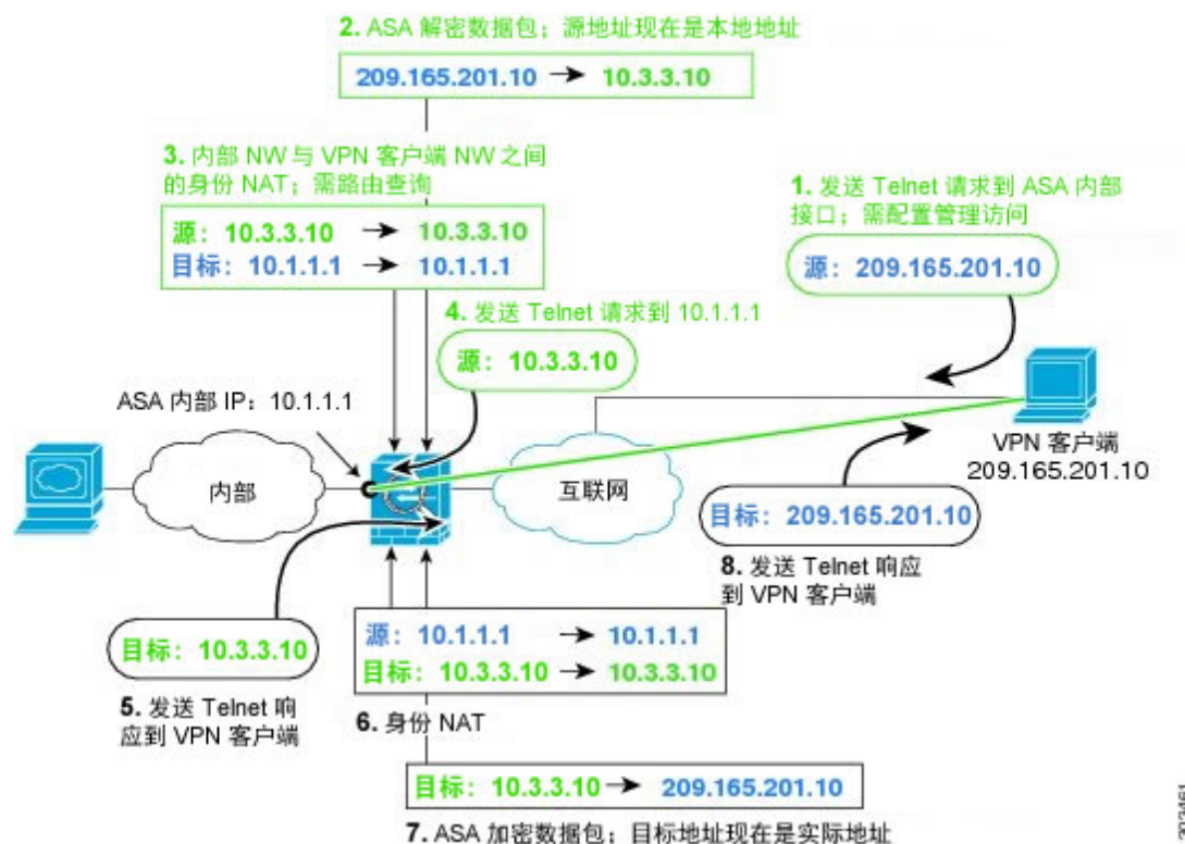
图 43: VPN 管理访问
