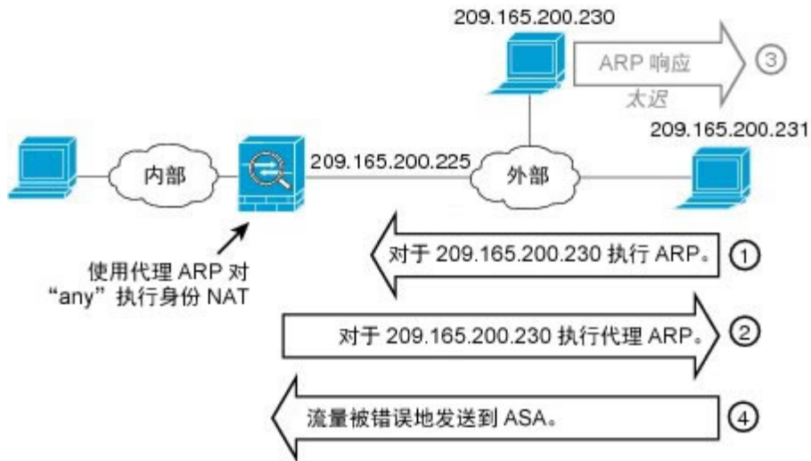
图 36: 身份 NAT 的代理 ARP 问题
