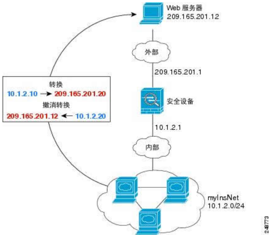
图 28: 面向内部 Web 服务器的动态 NAT，面向外部 Web 服务器的静态 NAT
