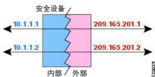
图 20: 静态 NAT
