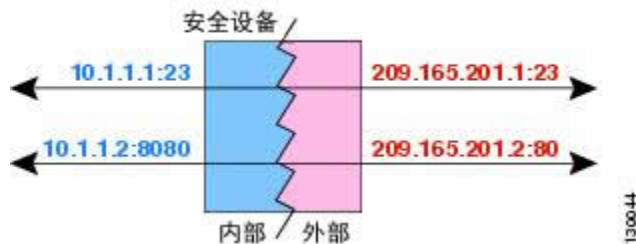
图 21: 支持端口转换的典型静态 NAT 场景
