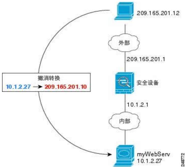
图 27: 面向内部 Web 服务器的静态 NAT
