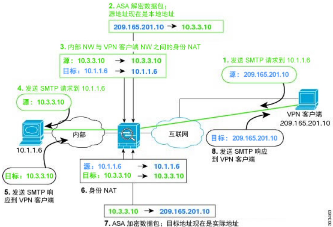
图 40: 面向 VPN 客户端的身份 NAT
