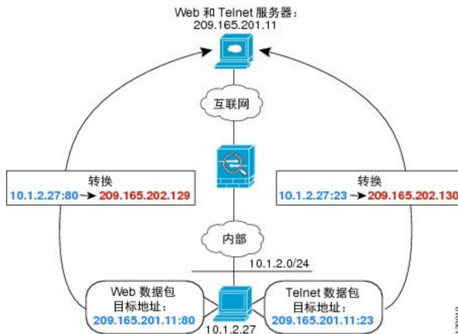
图 32: 使用不同目标端口的两次 NAT
