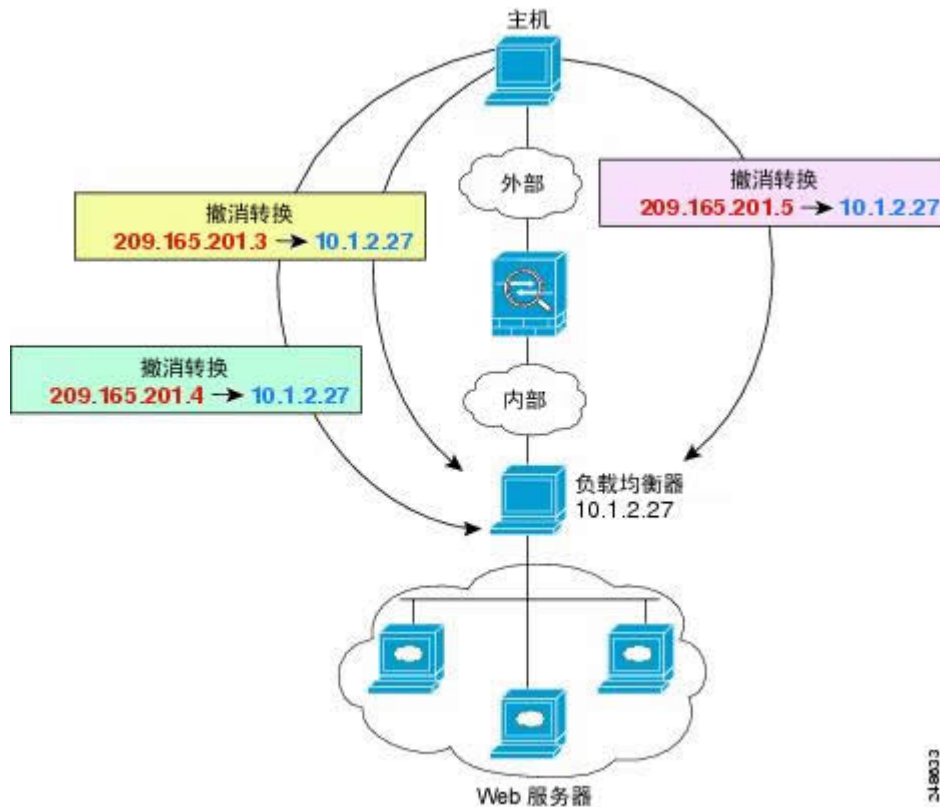
图 29: 内部负载均衡器的一对多静态 NAT
