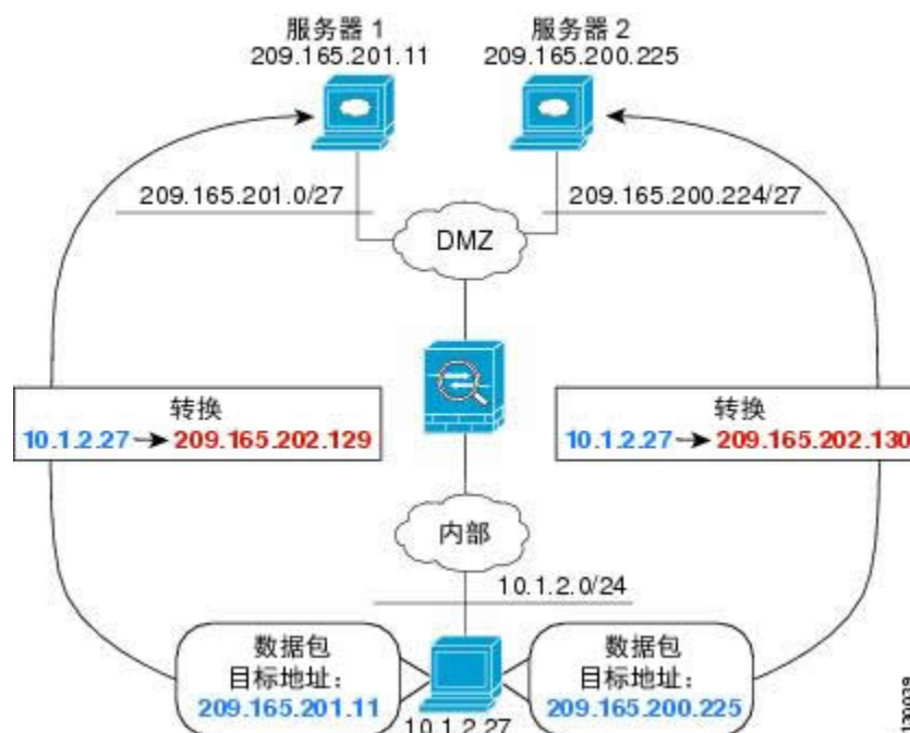
图 31: 使用不同目标地址的两次 NAT
