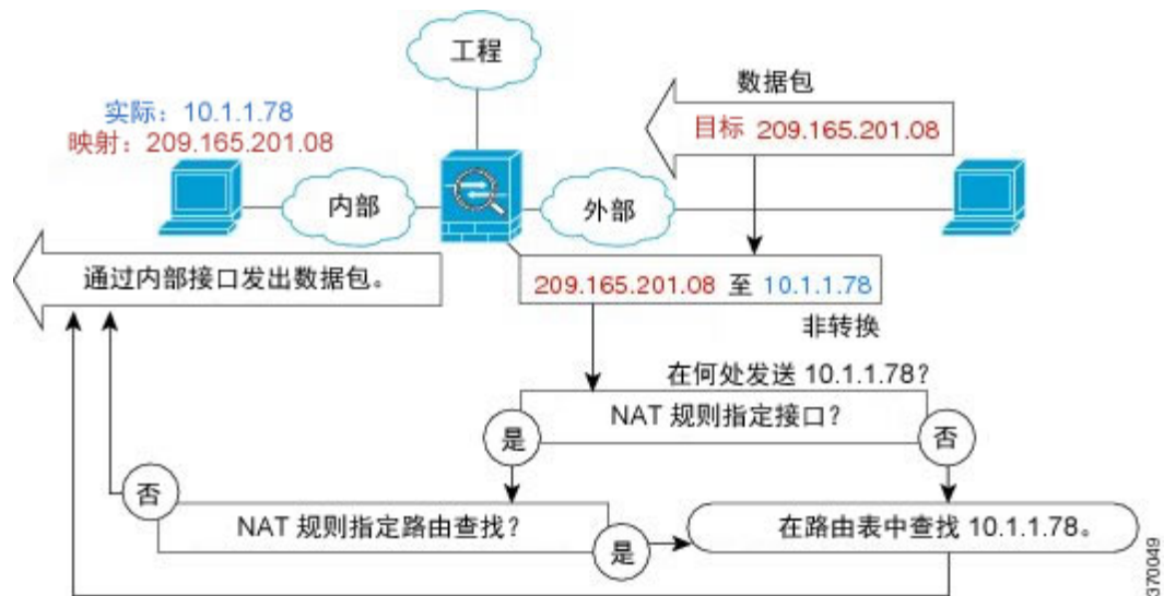
图 38: 含 NAT 的路由模式出口接口选择
