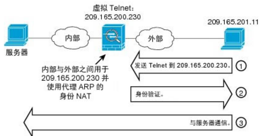
图 37: 代理 ARP 和虚拟 Telnet
