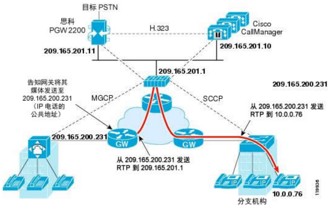
图 46: 配合使用 NAT 与 MGCP
