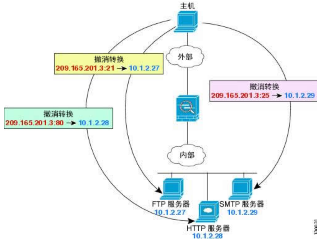
图 30: 支持端口转换的静态 NAT
