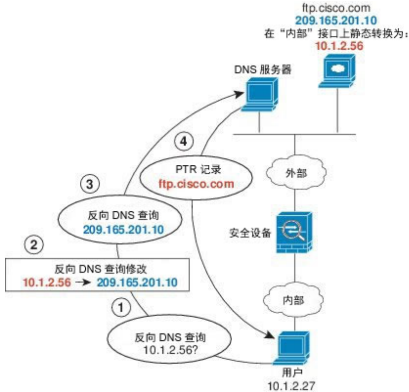
图 45: PTR 修改，主机网络上的 DNS 服务器
