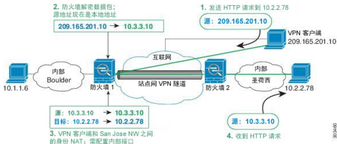
图 42: VPN 客户端访问站点到站点 VPN
