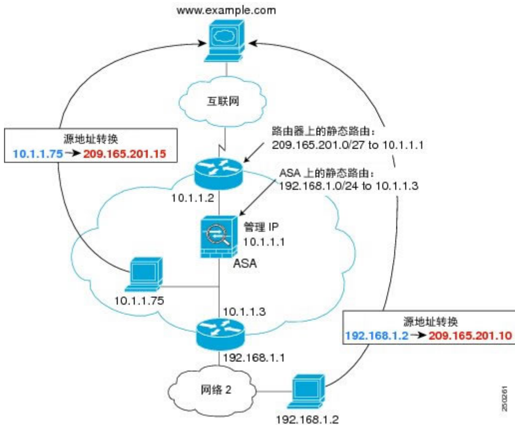
图 35: NAT 示例: 透明模式
