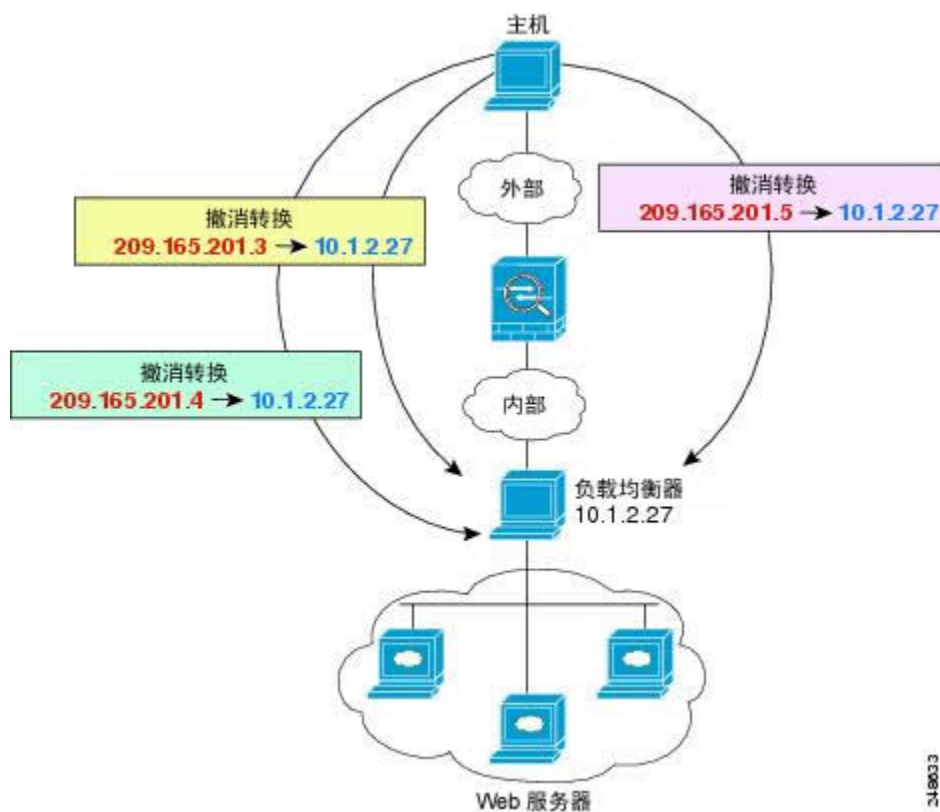
图 23: 一对多静态 NAT 示例
