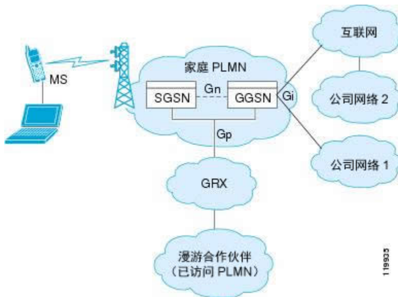
图 47: GPRS 隧道协议
