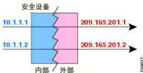
图 17: 动态 NAT
