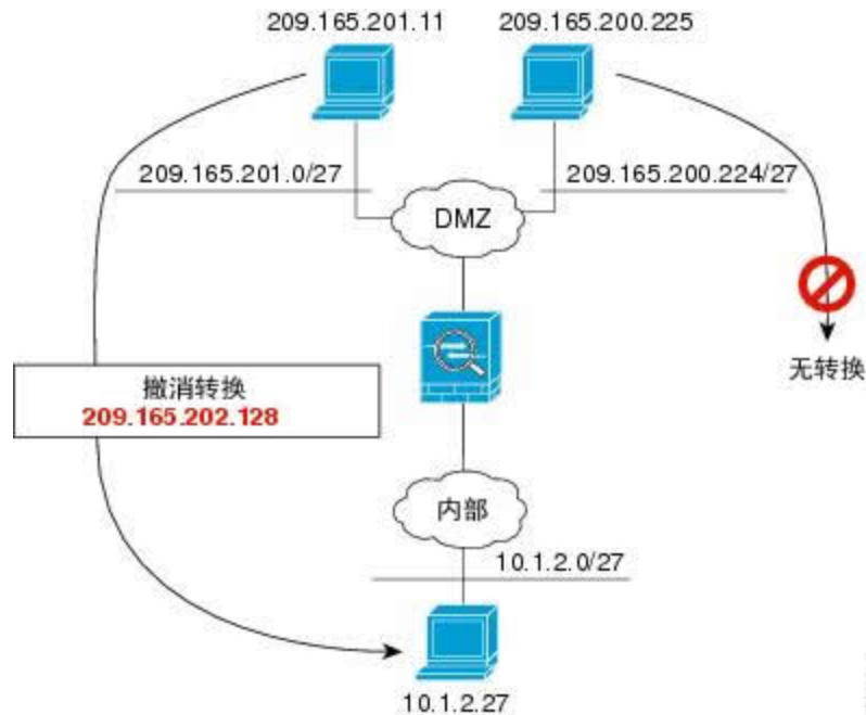
图 33: 支持目标地址转换的两次静态 NAT
