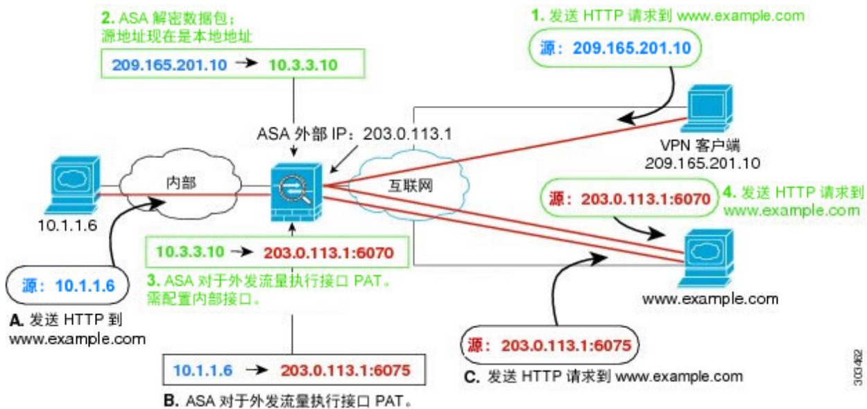
图 39: 面向互联网绑定 VPN 流量的接口 PAT (接口内)
