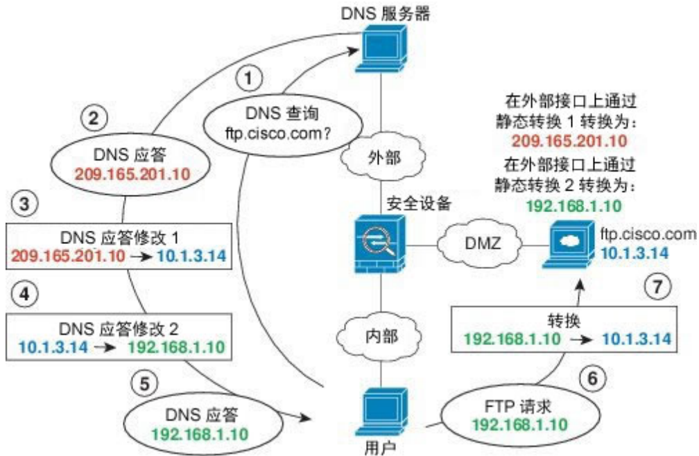
图 44: 独立网络上的 DNS 应答修改、DNS 服务器、主机和服务器
